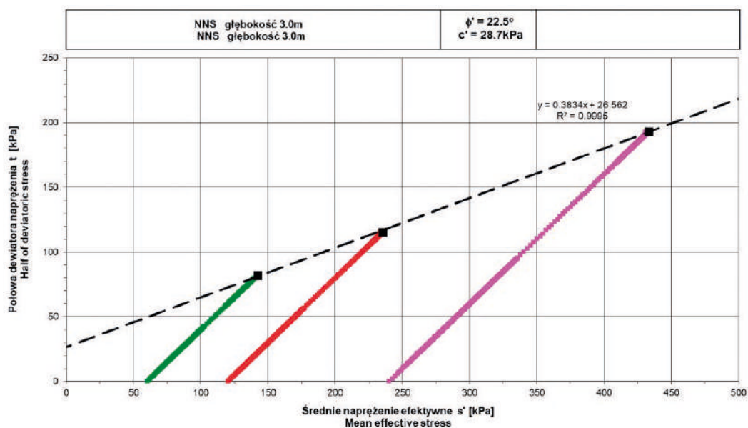
Rys. 9. Wyniki badań w aparacie trójsiowym TX CID serii H [3]
