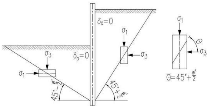
Rys. 6 Orientacja naprężeń głównych względem płaszczyzn poślizgu oraz w próbce gruntu badanej w aparacie trójsiowym
