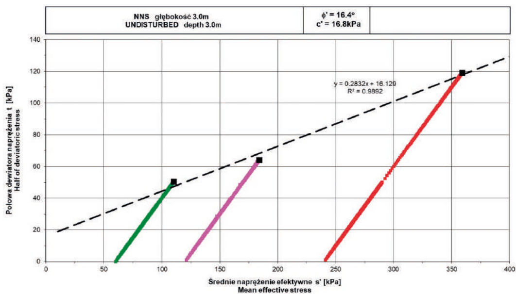
Rys. 8. Wyniki badań w aparacie trójsiowym TX CID serii V [3]
